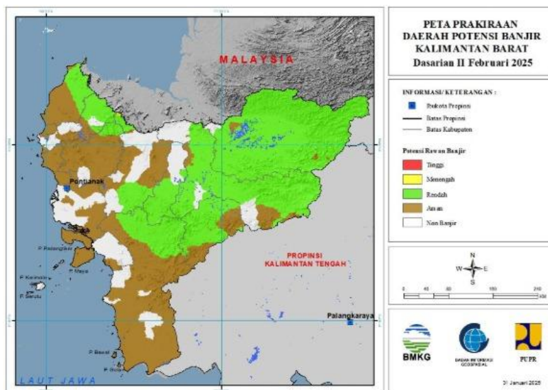
Gambar 15. Peta Potensi Banjir Dasarian II Bulan Februari 2025
